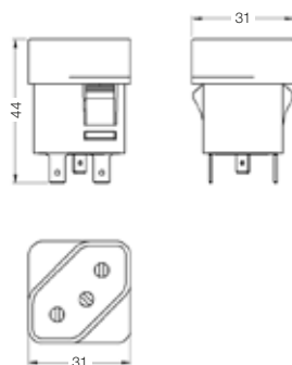
Tomada de painel quadrada colar externo (faston)
