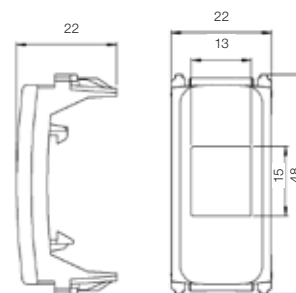
Módulo tomada RJ 45
