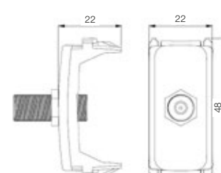
Tomada para antena
