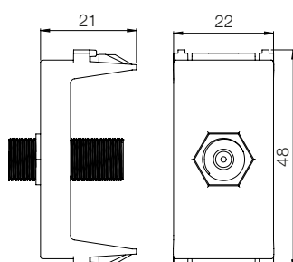
Módulo antena
