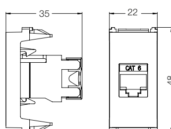
Módulo RJ45 CAT6
