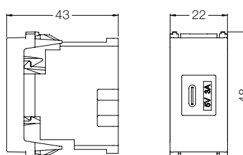
Módulo carregador keystone USB tipo-C
