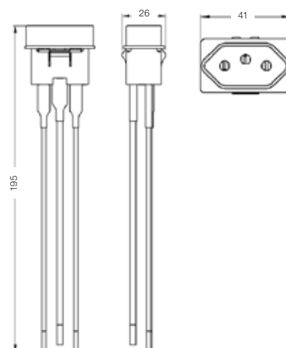
Tomada de painel retangular colar interno (cabo)
