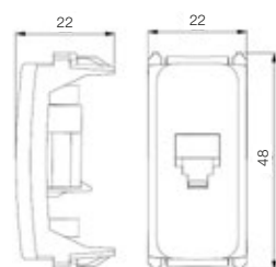
Tomada RJ11
