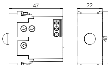
Módulo sensor de presença
