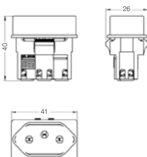
Tomada de painel retangular colar externo (parafuso)
