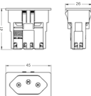
Tomada de painel retangular colar interno (parafuso)
