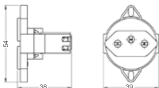
Tomada de piso (aba curta)
