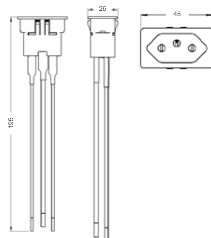
Tomada de painel retangular colar interno (cabo)
