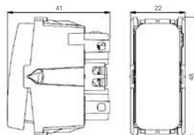
Pulsador universal sem gravação
