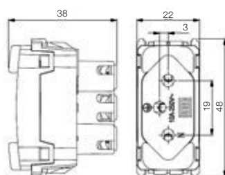
Tomada 2P+T-10 A
