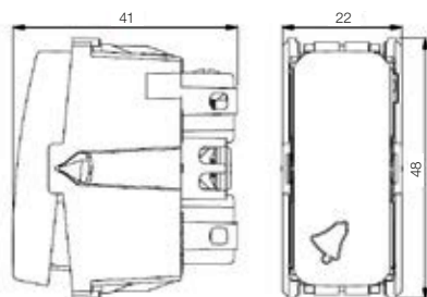
Pulsador campainha
