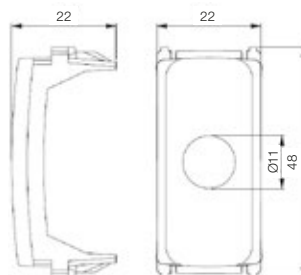
Módulo saída de fio
