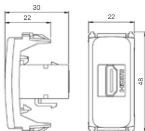
Tomada HDMI
