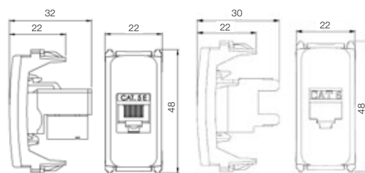
Tomada RJ45 CAT 5E/CAT 6
