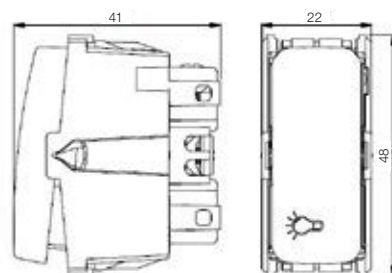
Pulsador minuteria
