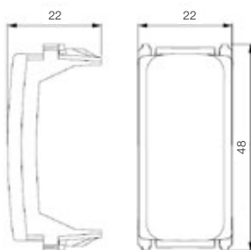
Módulo cego
