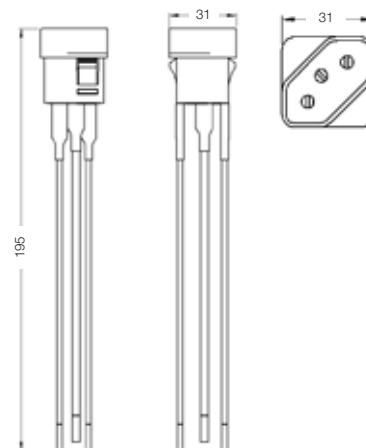
Tomada de painel retangular colar externo (cabo)
