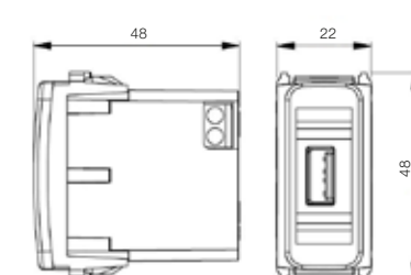
Tomada USB
