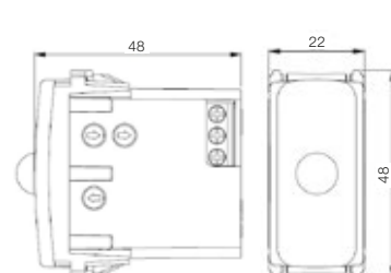
Sensor de presença
