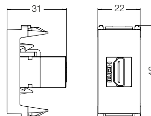
Módulo HDMI
