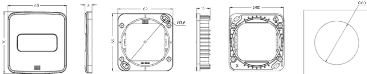
Furação
