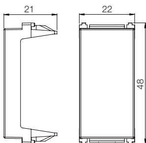
Módulo cego
