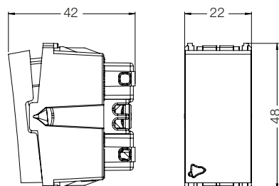
Pulsador campainha
